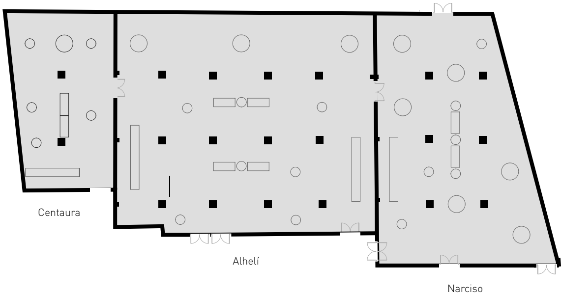
Disposición de mesas para Cóctel según normativa CTE-DB SI
